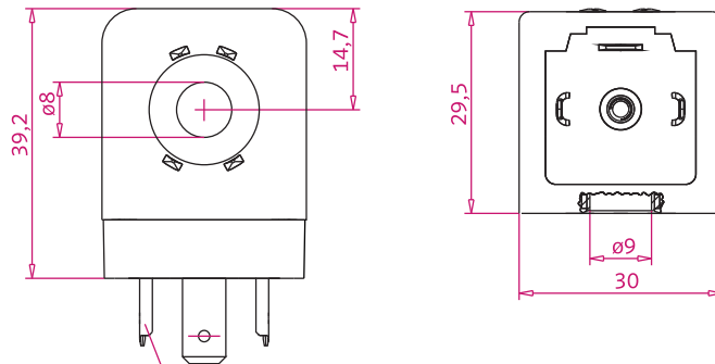
Electrical Connection DIN EN 175301-803-A/ISO 4400
